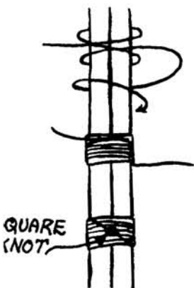
SHORT SEIZING
